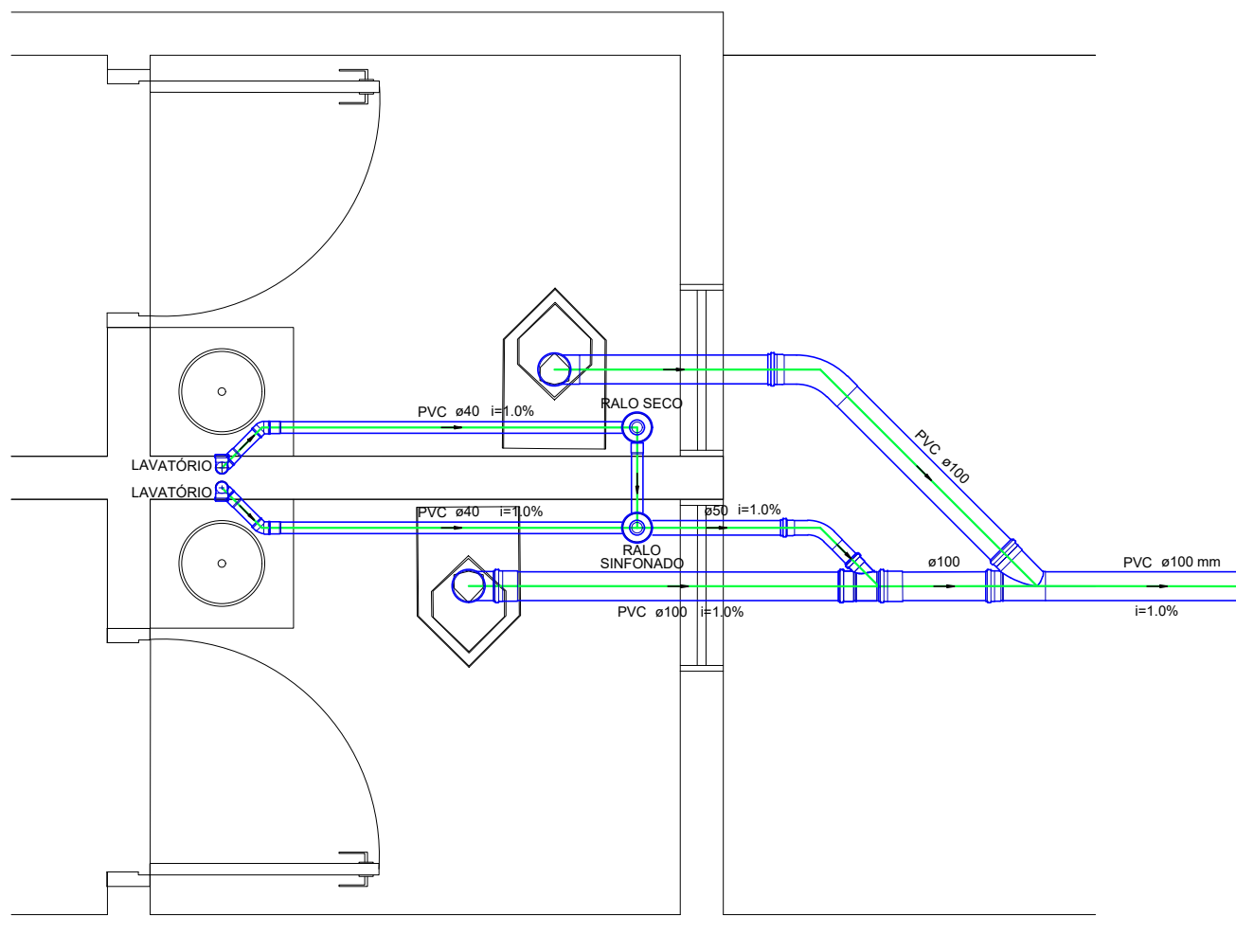
Detalhe Banheiros Administração Escala 1:25
